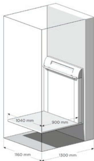
900 x 1040
